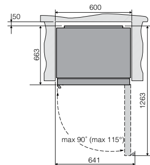
Dimensions encastrement
